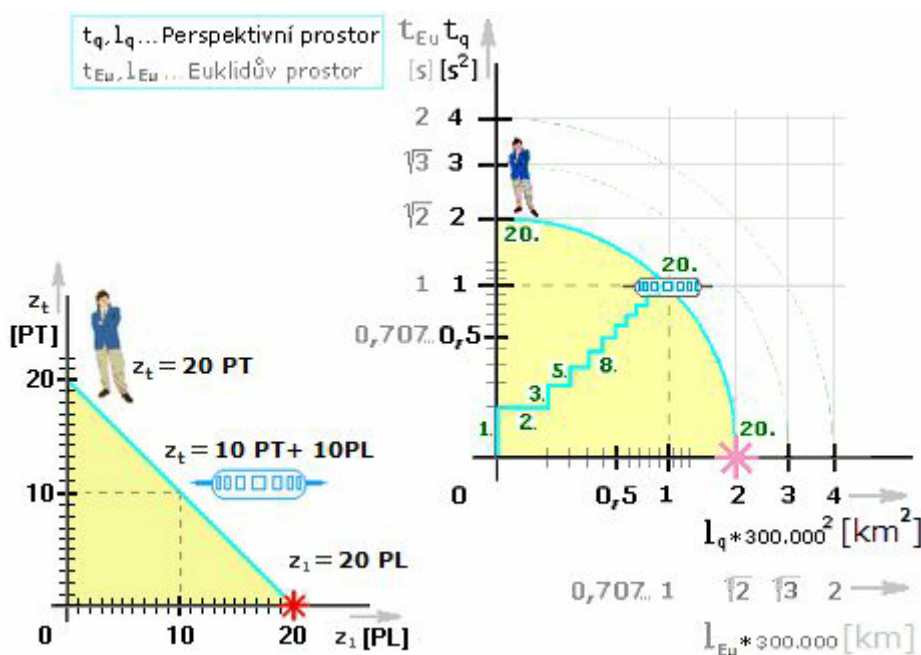
Obr. 18. Stav ve 20. pulsu. Vlevo diskretní prostor. Vpravo Euklidův a perspektivní prostor, s vodorovnou osou, značenou násobky délkové jednotky.
