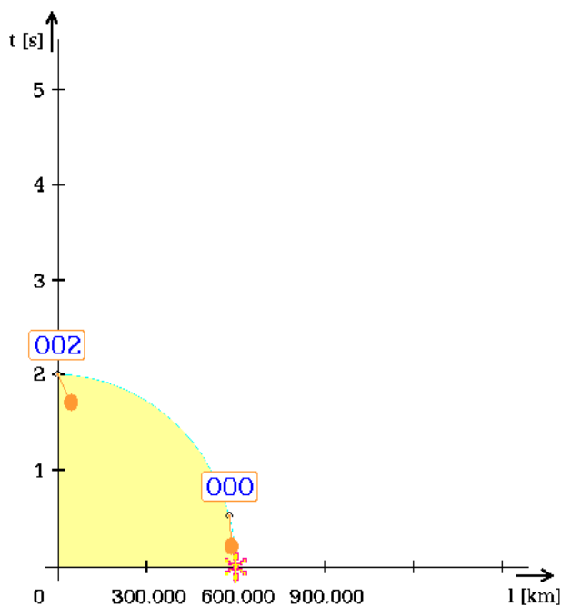
Obr. 5. Kyvadlové hodiny v souměrném grafu časoprostoru
