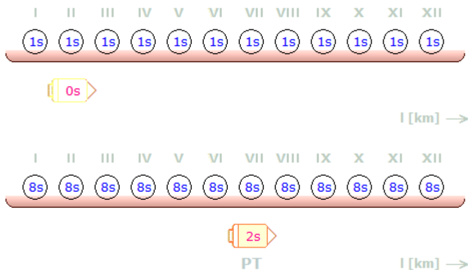
Obr. 16. Koráb ověřuje Lorentzův čas
