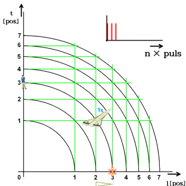
Obr. 13. Dvojrzměrný časoprostor. Zelená síť zdůrazňuje souvislost perspektivního prostoru s diskrétním
