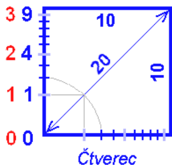
Obr. 12. Matematizace perspektivního prostoru
